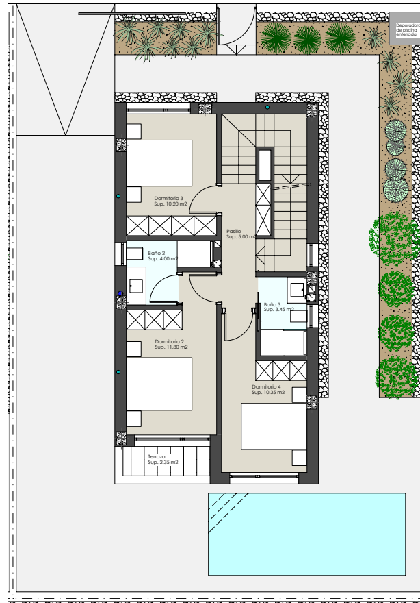
Planta primera
