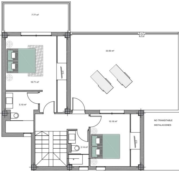
PLANTA PRIMERA
